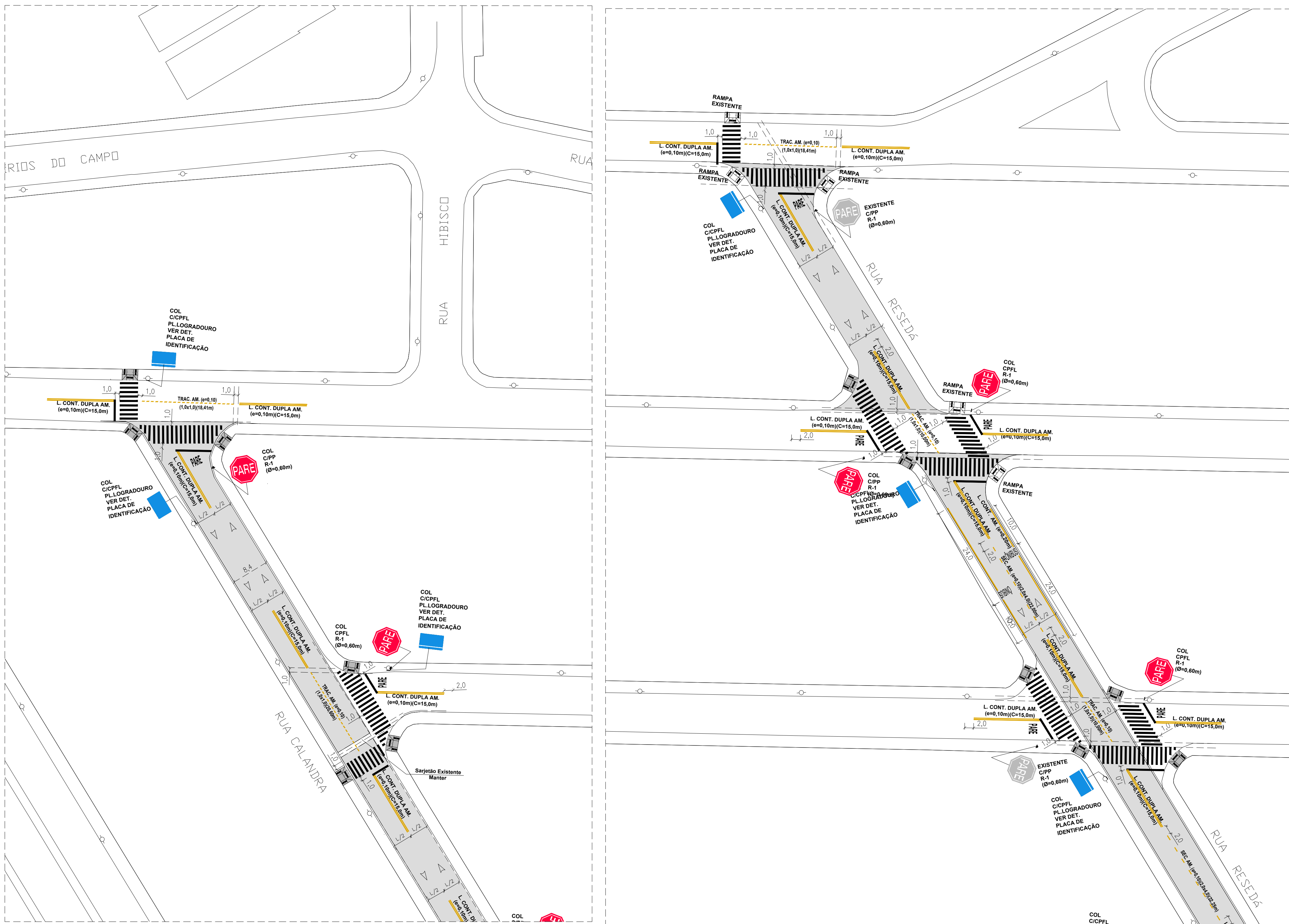
SINALIZAÇÃO HORIZONTAL E VERTICAL Escala: 1:500 DETALHE 02
